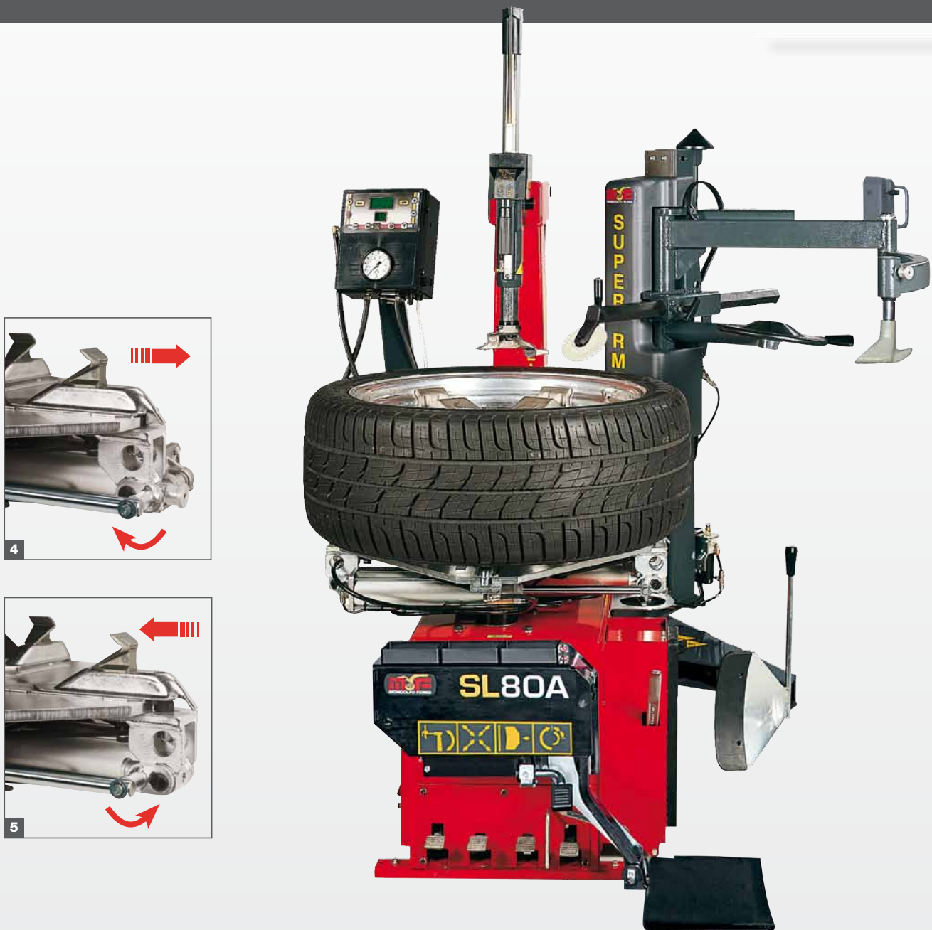
Foto AS 944 completa degli optional SUPER RM NEW , RM2, RM3, Airtronic e del sollevatore ruota SL80 A. Photo of AS944 complete with optional accessories SUPER RM NEW , RM2, RM3, Airtronic and the wheel lifter SL80 A.
